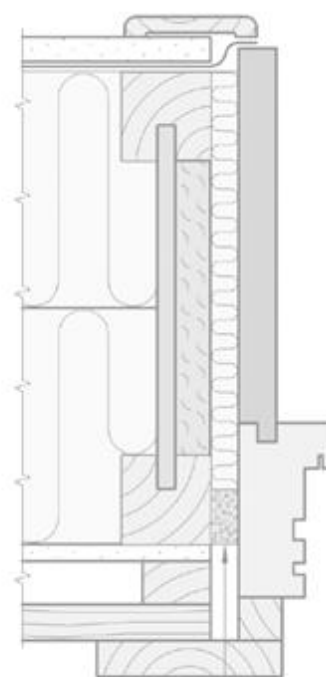
Ekspanderende fugebånd
