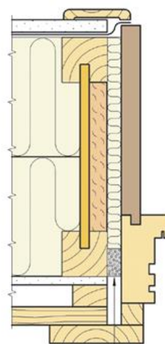
Ekspanderende fugebånd
